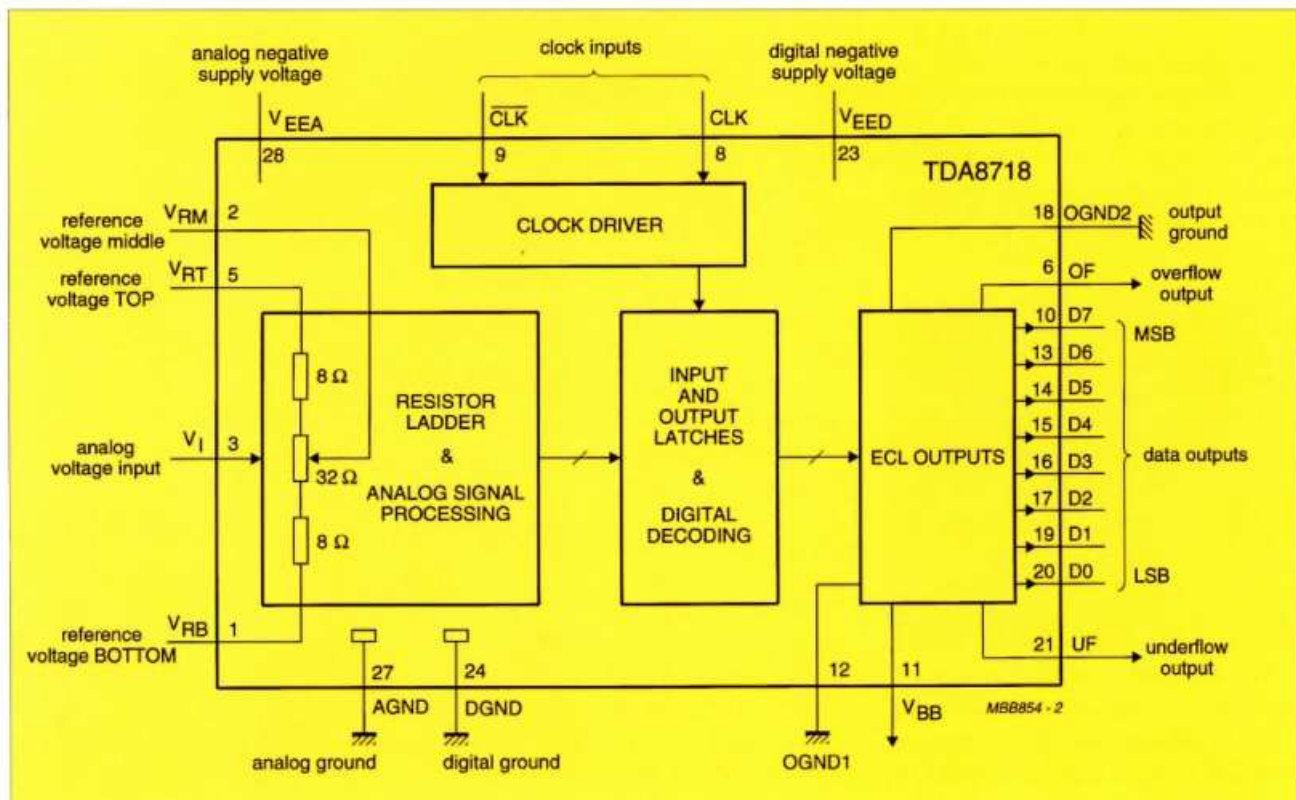
Blokschema van de ultrasnelle 8-bit A/D converter TDA 8718.
